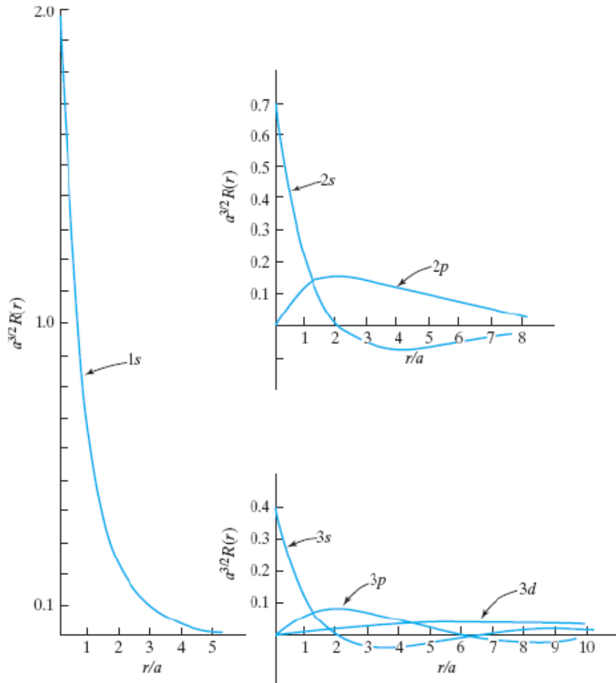
氢原子 ( Z = 1 ) 波函数径向因子 R_{nl}(r) 的示意
